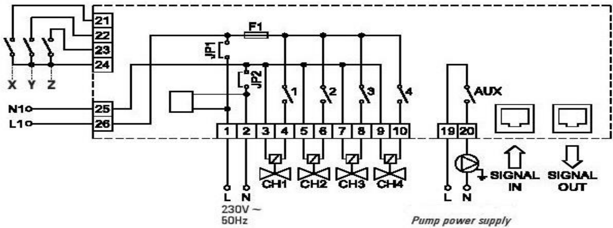
Fig. 4: Inkopplingschema
