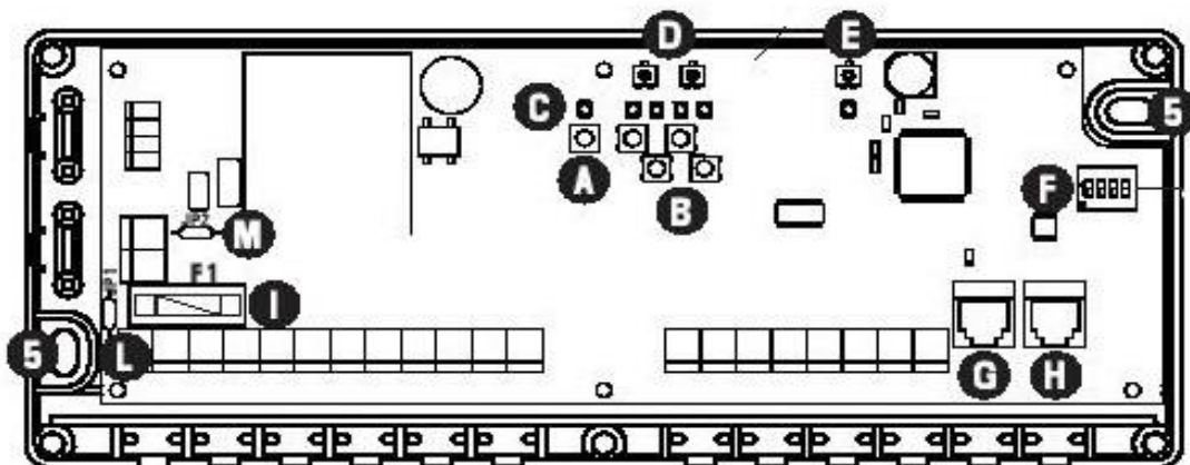
Fig. 2: Utstyringsenhetens kretskort, med dess byglar, säkring, DIP-switchar, etc.
